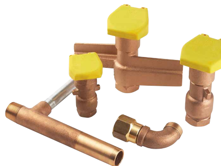
Быстродействующие клапаны
