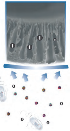
Фрагмент волокна Hollow fiber section
