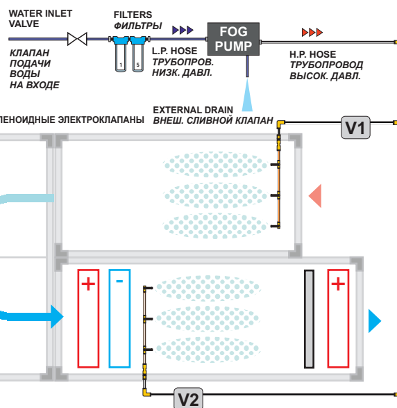
Типичная схема монтажа АКВ: Увлажнение и предварительное охлаждение AHU Mounting layout example: Humidification and Pre-cooling
